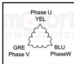
Wiring cable
