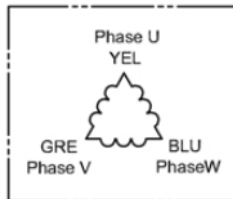
Wiring cable
